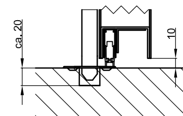
absenkbare Bodendichtung
