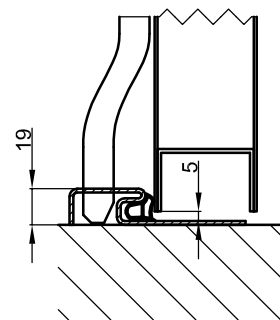
untere Anschlagdichtung
