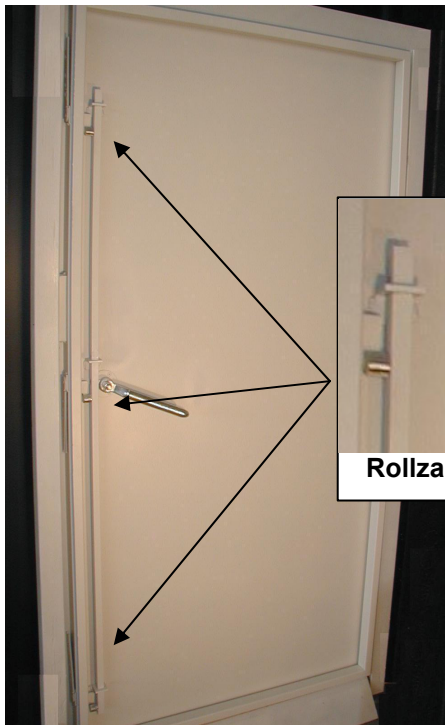
Beidseitig bedienbarer Presshebel mit Verriegelungs- stange und 3 Rollzapfen
